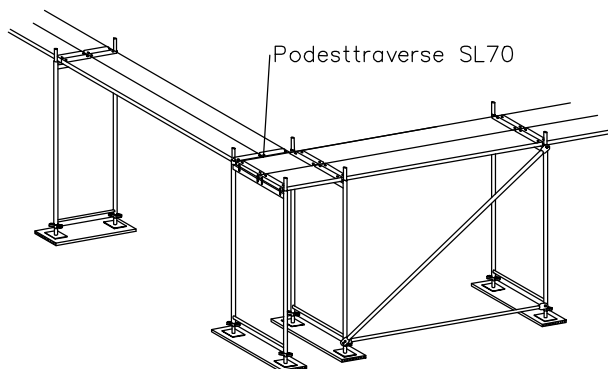
Bild 7: Eckausbildung (Variante 2)
