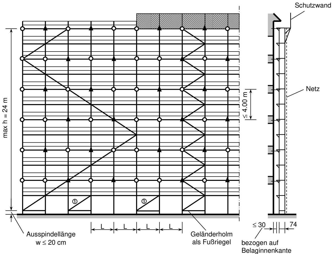
Bild 41: Gerüst mit Netzbekleidung vor teilweise offener Fassade Ankerraster: 4 m
