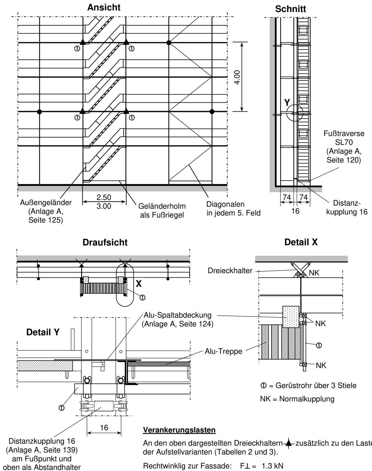
Bild 60: Gleichläufiger Treppenaufstieg
