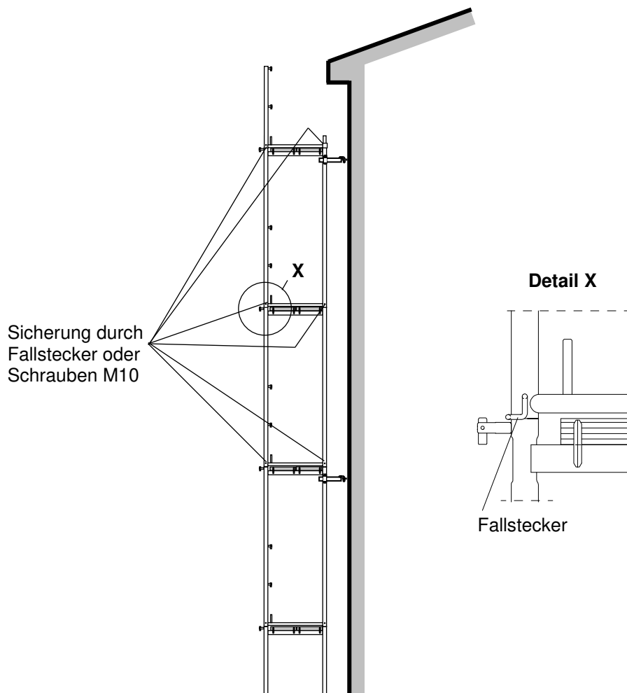
Bild 56: Zugfeste Verbindung des Gerüsts
