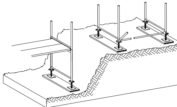
Bild 2: Ausgleichsrahmen
