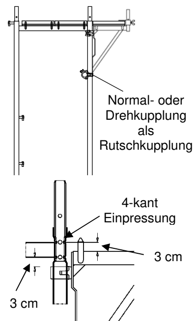
Bild 24: Konsole 64
