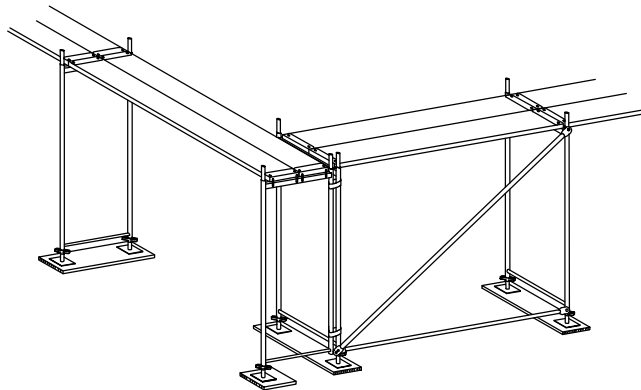
Bild 6: Eckausbildung (Variante 1)
