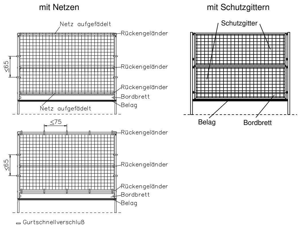
Bild 28: Schutzwand
